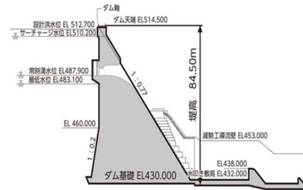
堤体断面図
