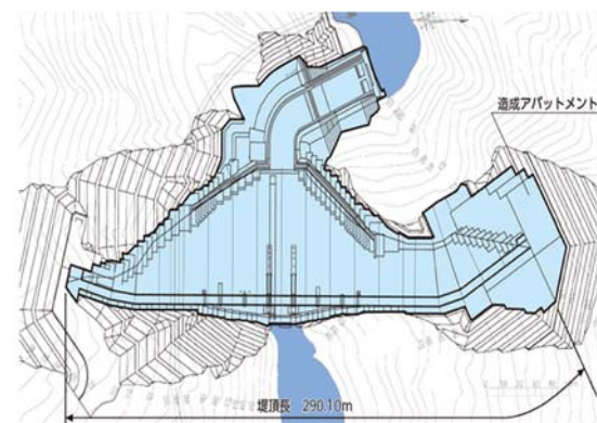
堤体平面図
