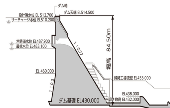
堤体断面図
