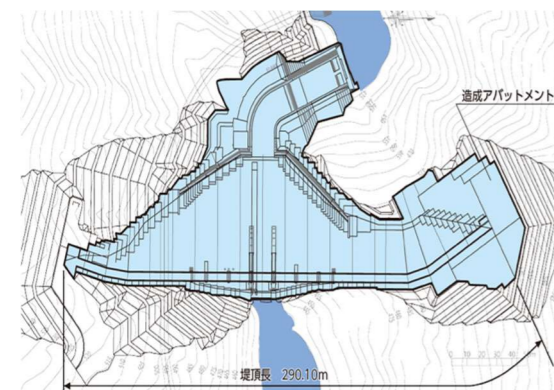
堤体平面図
