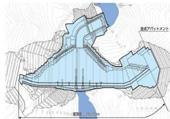
堤体平面図
