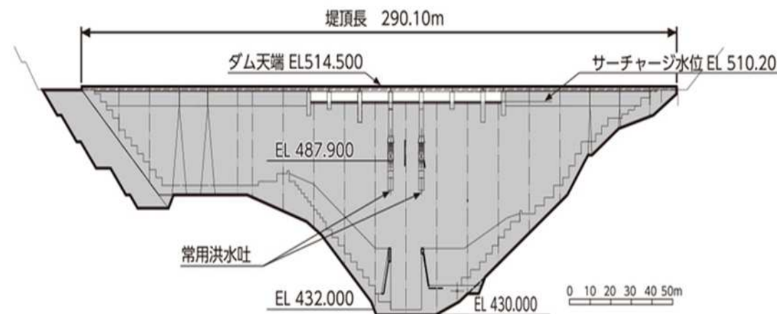
堤体下流面図
