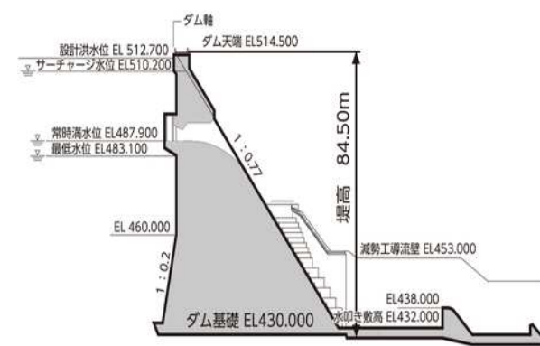
堤体断面図
