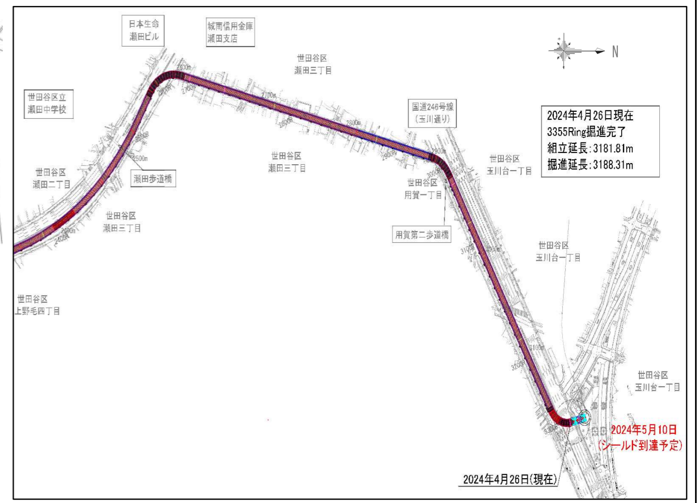
シールド掘進状況
