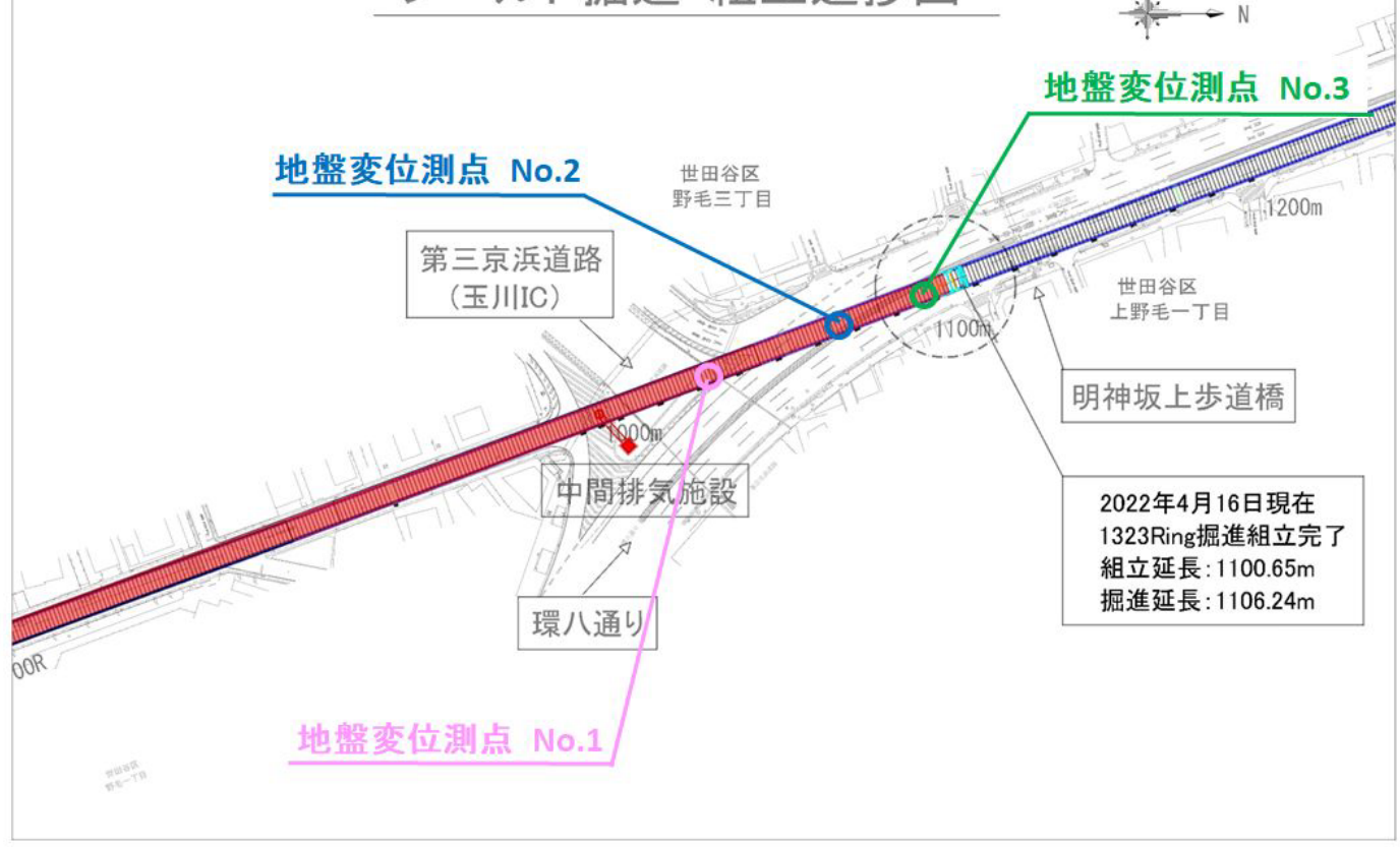
地盤変位量推移 2022年4月1日～2022年4月15日
