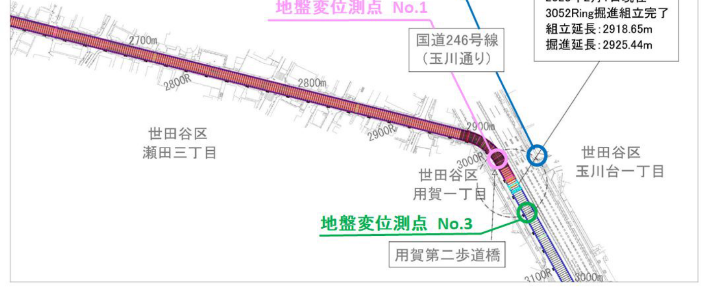
地盤変位量推移 2023年1月16日～2023年1月31日
