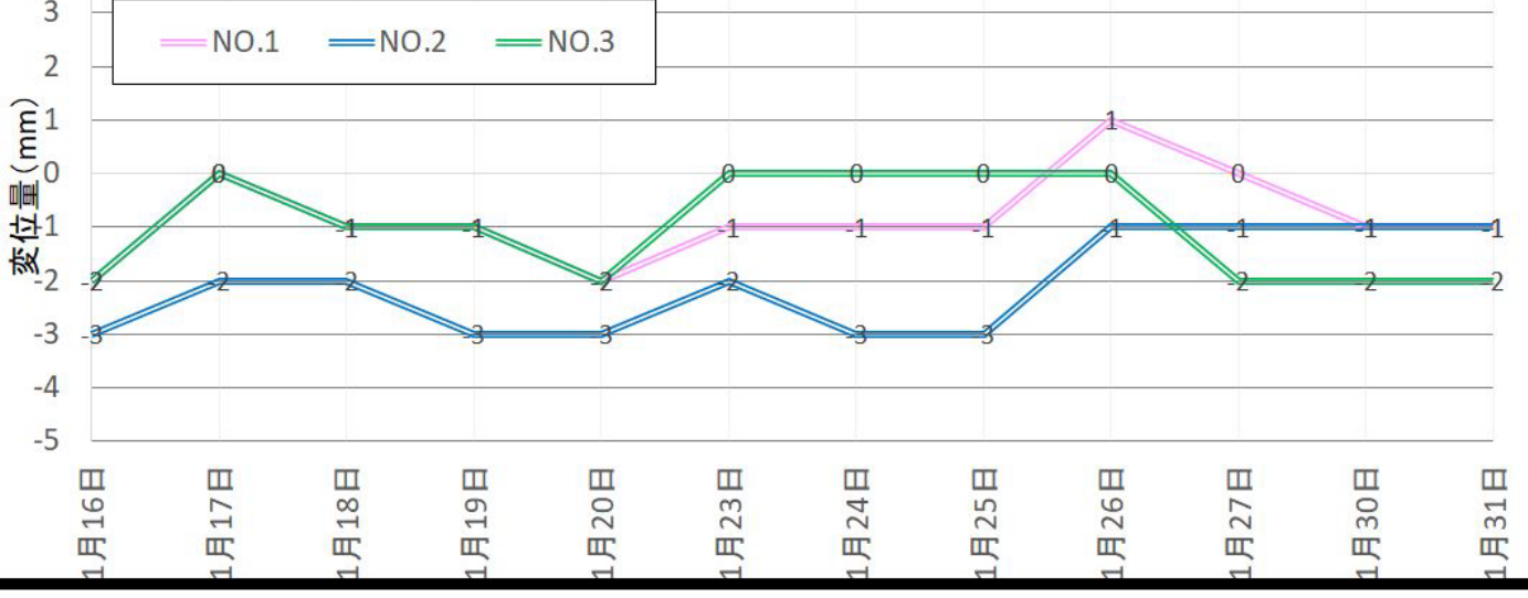
地盤変位量推移 2023年1月16日～2023年1月31日
