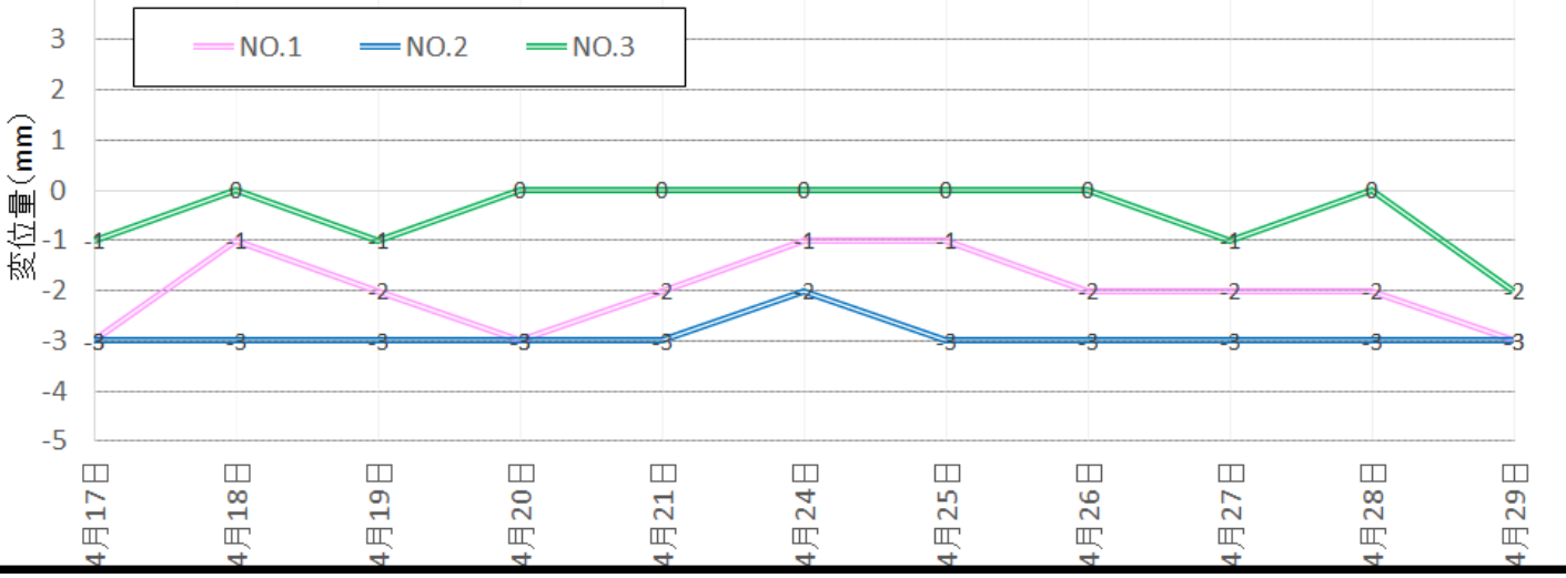
地盤変位量推移 2023年4月17日～2023年4月29日
