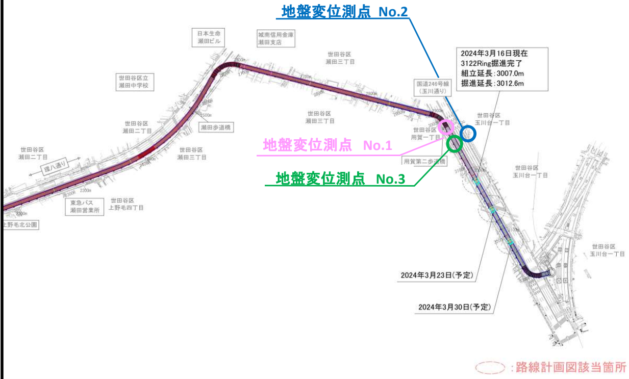
地盤変位量推移 2024年3月1日~2024年3月18日
